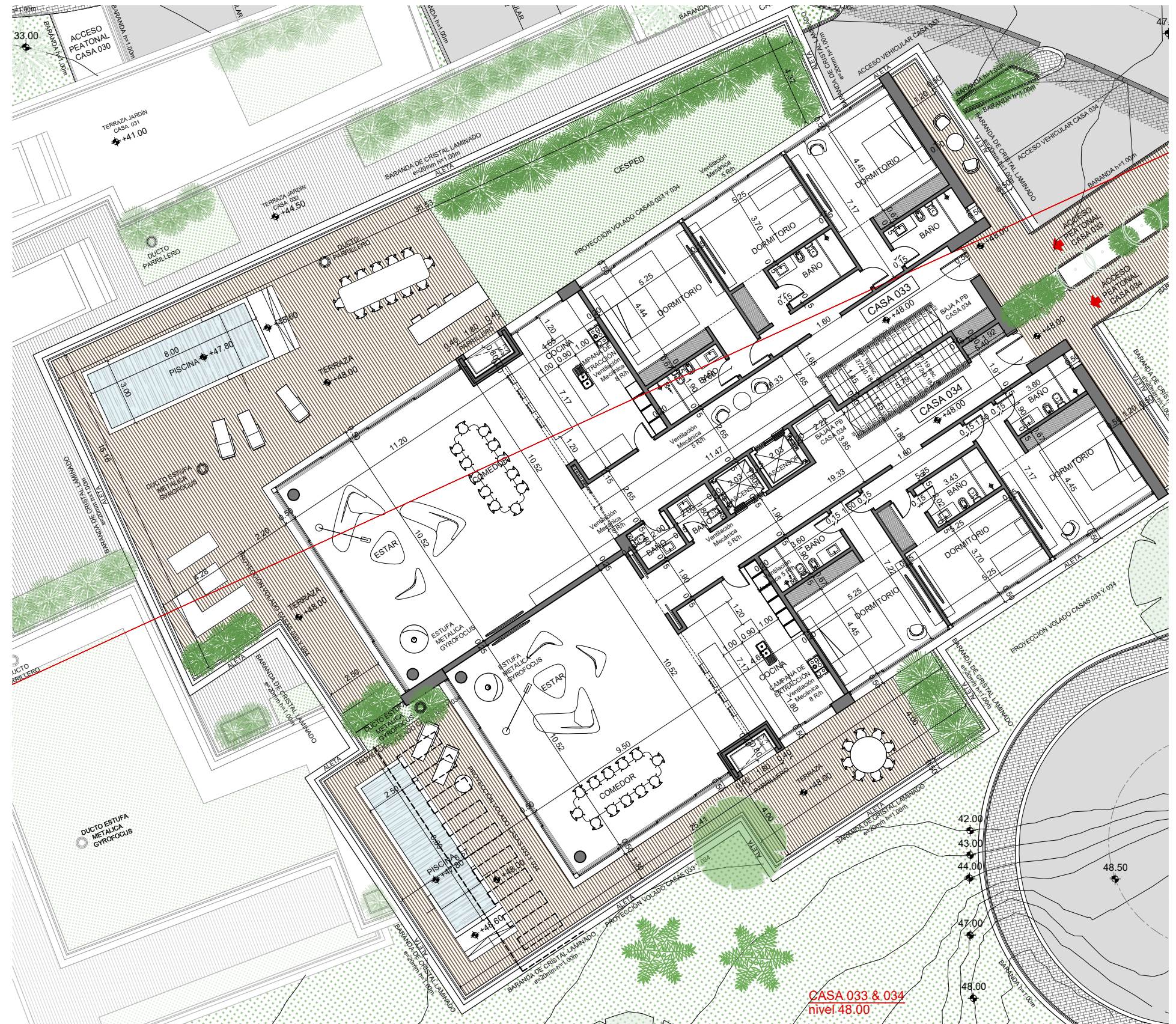
PLANTA NIVEL 02
