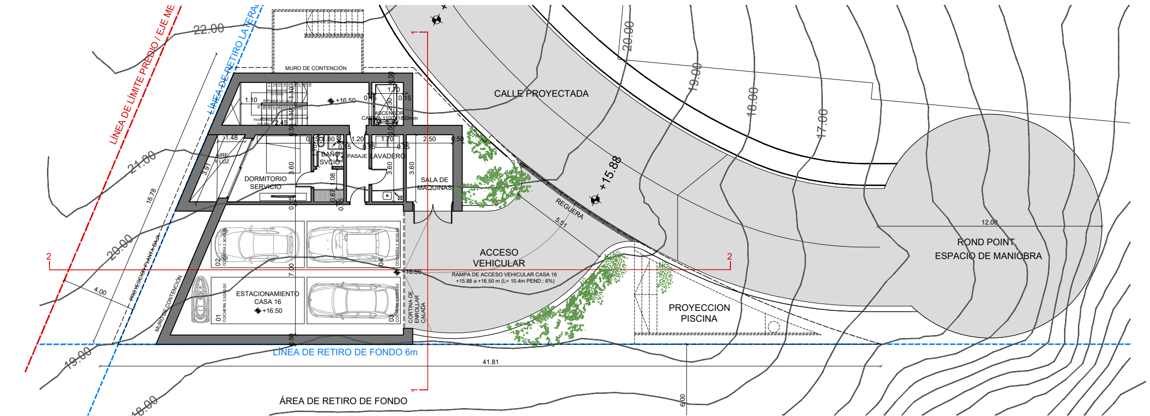
PLANTA NIVEL 01
