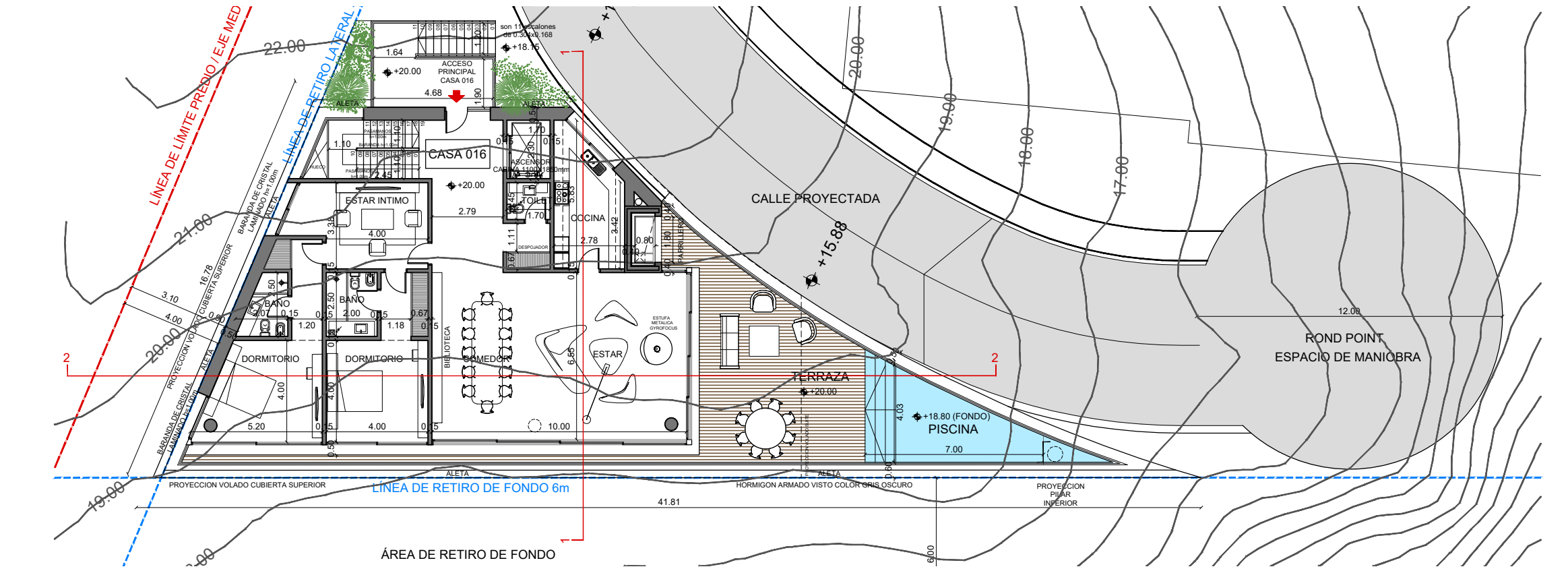
PLANTA NIVEL 02
