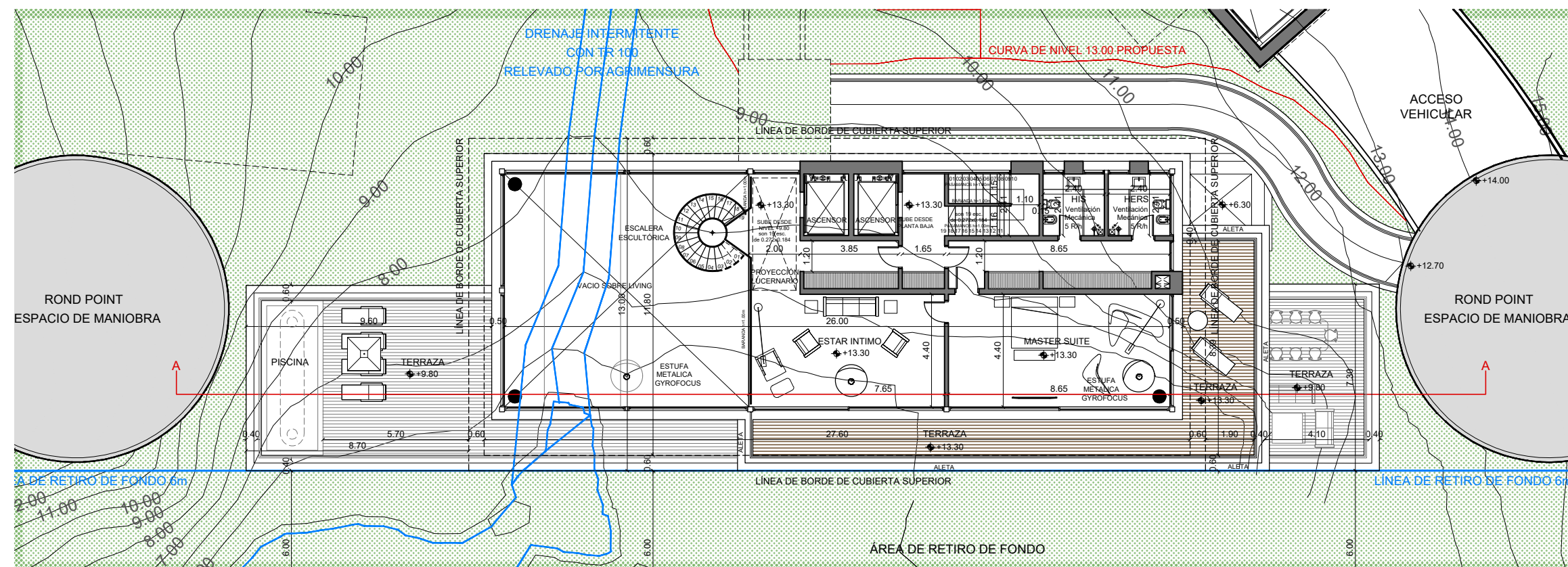
PLANTA NIVEL 04
