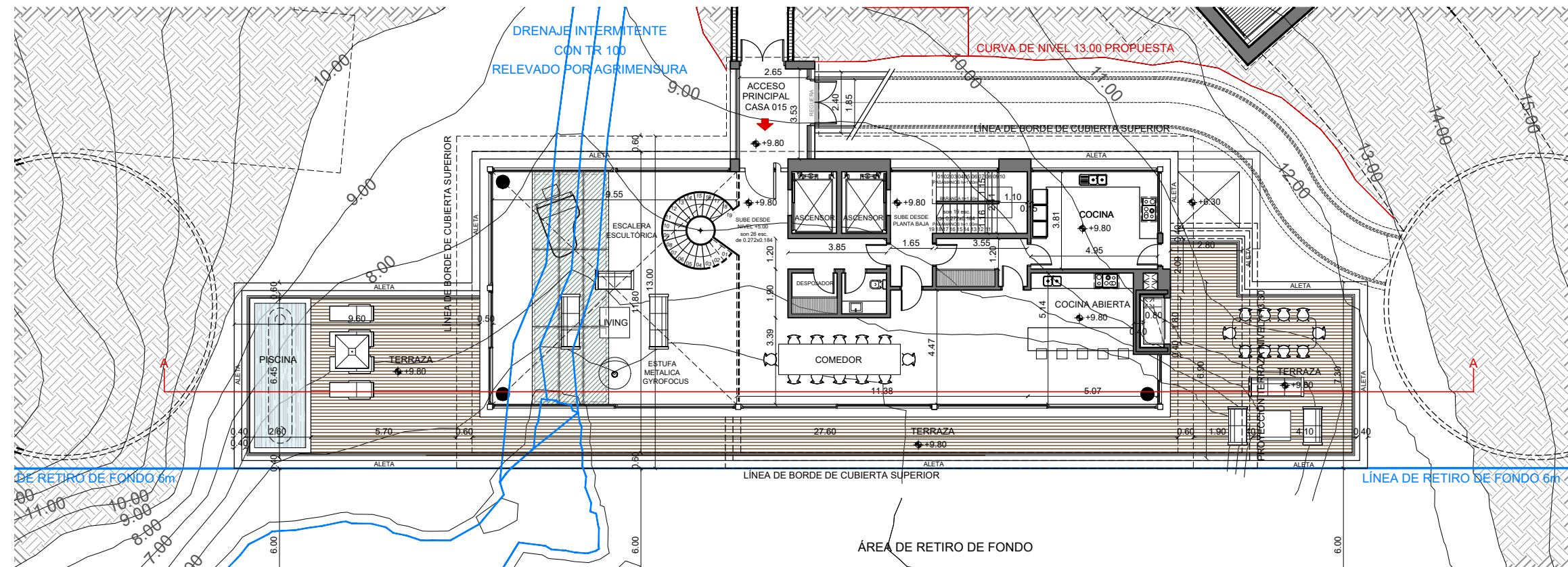
PLANTA NIVEL 03
