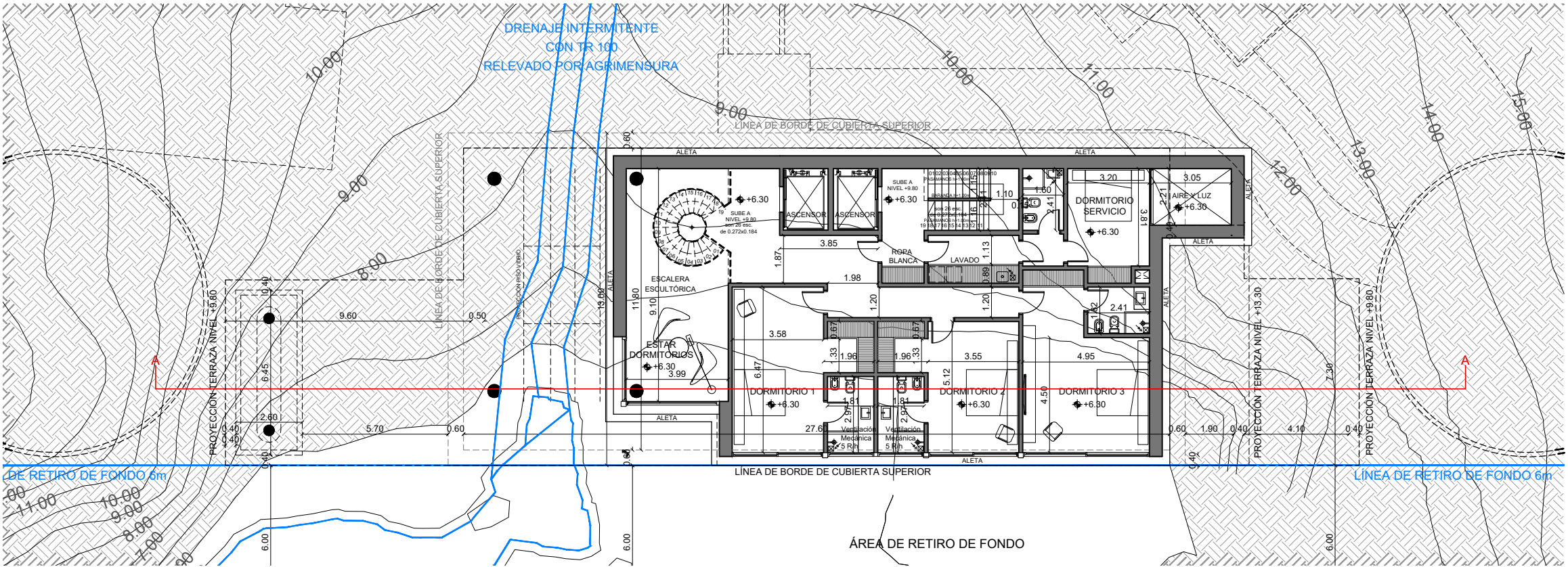
PLANTA NIVEL 02
