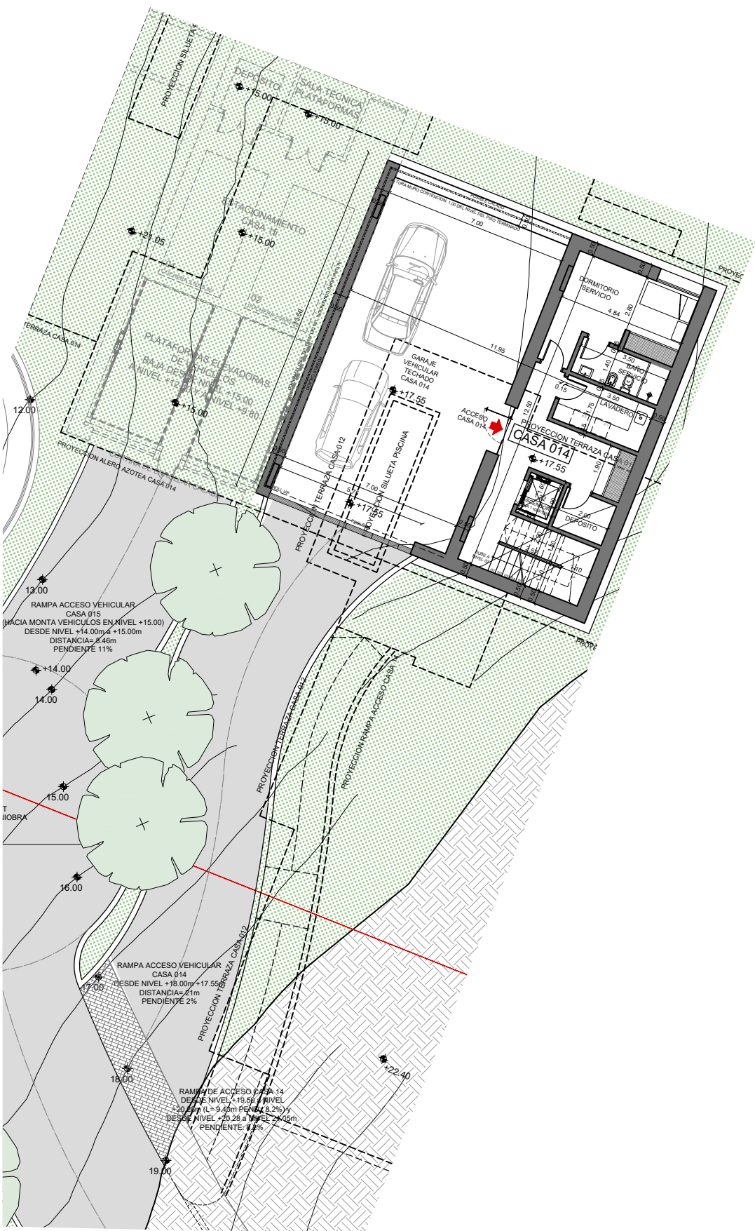
PLANTA NIVEL 01
