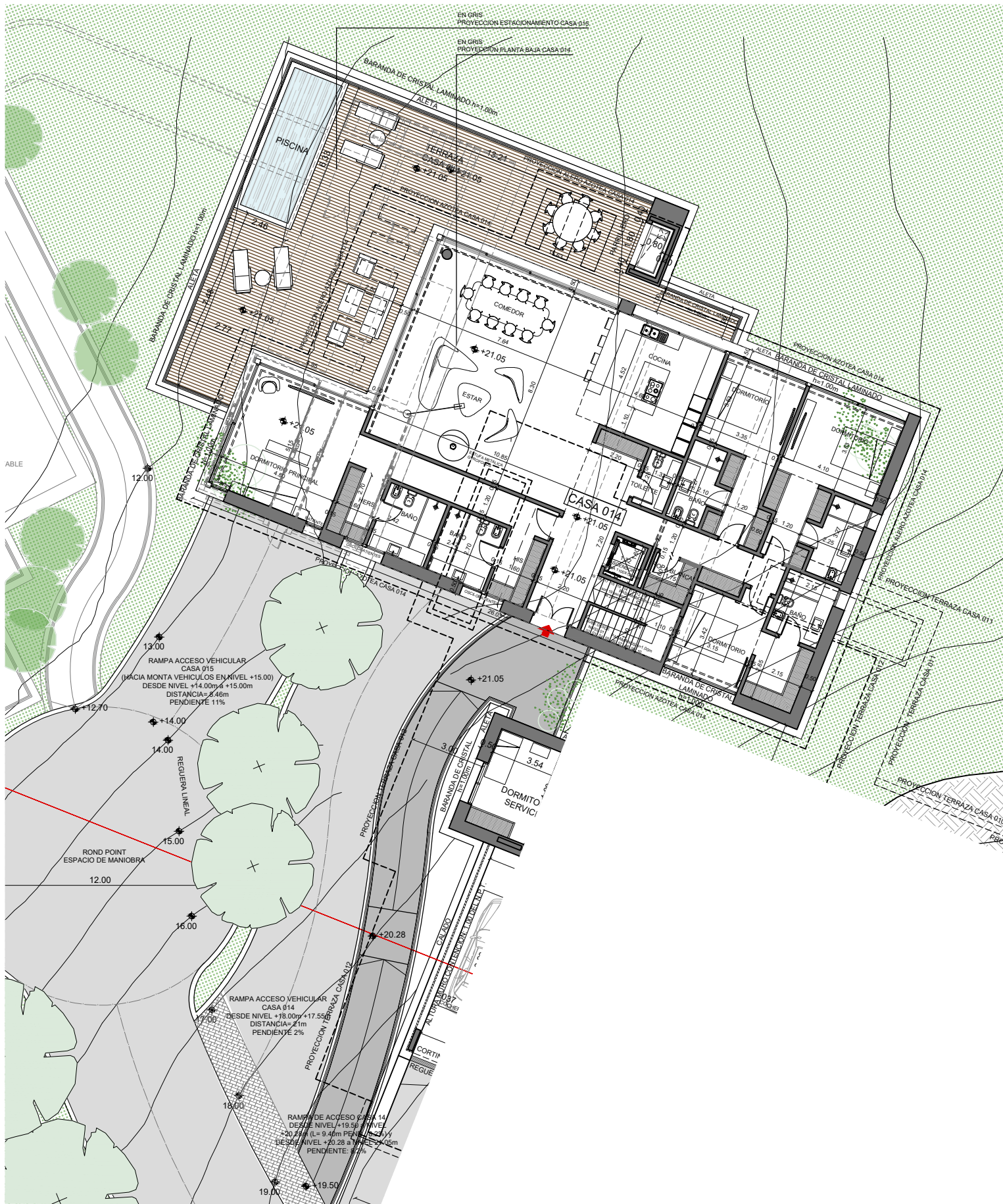
PLANTA NIVEL 02
