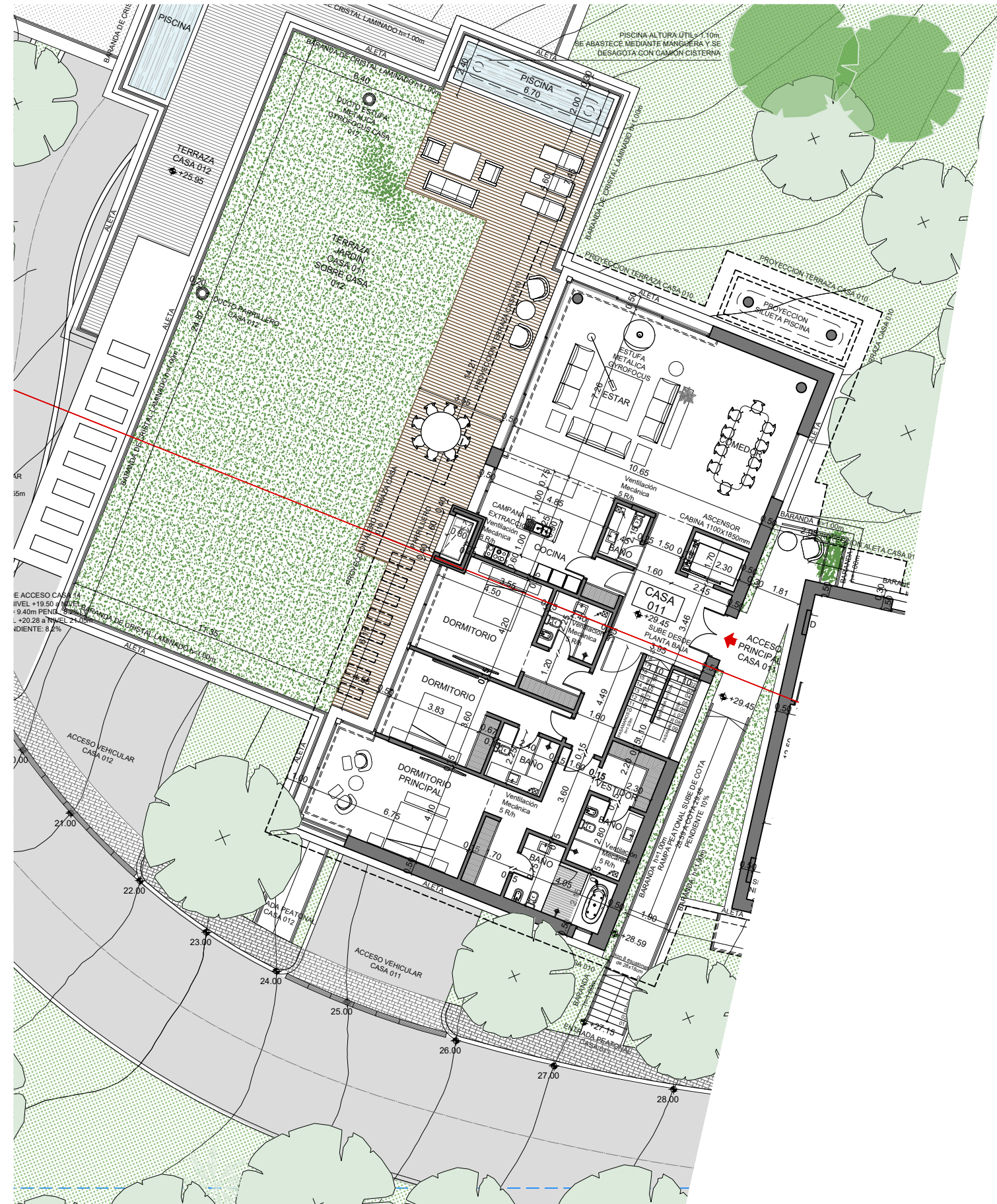
PLANTA NIVEL 02
