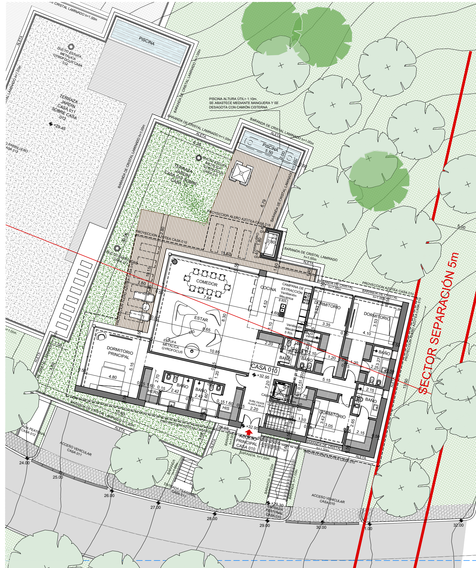
PLANTA NIVEL 02
