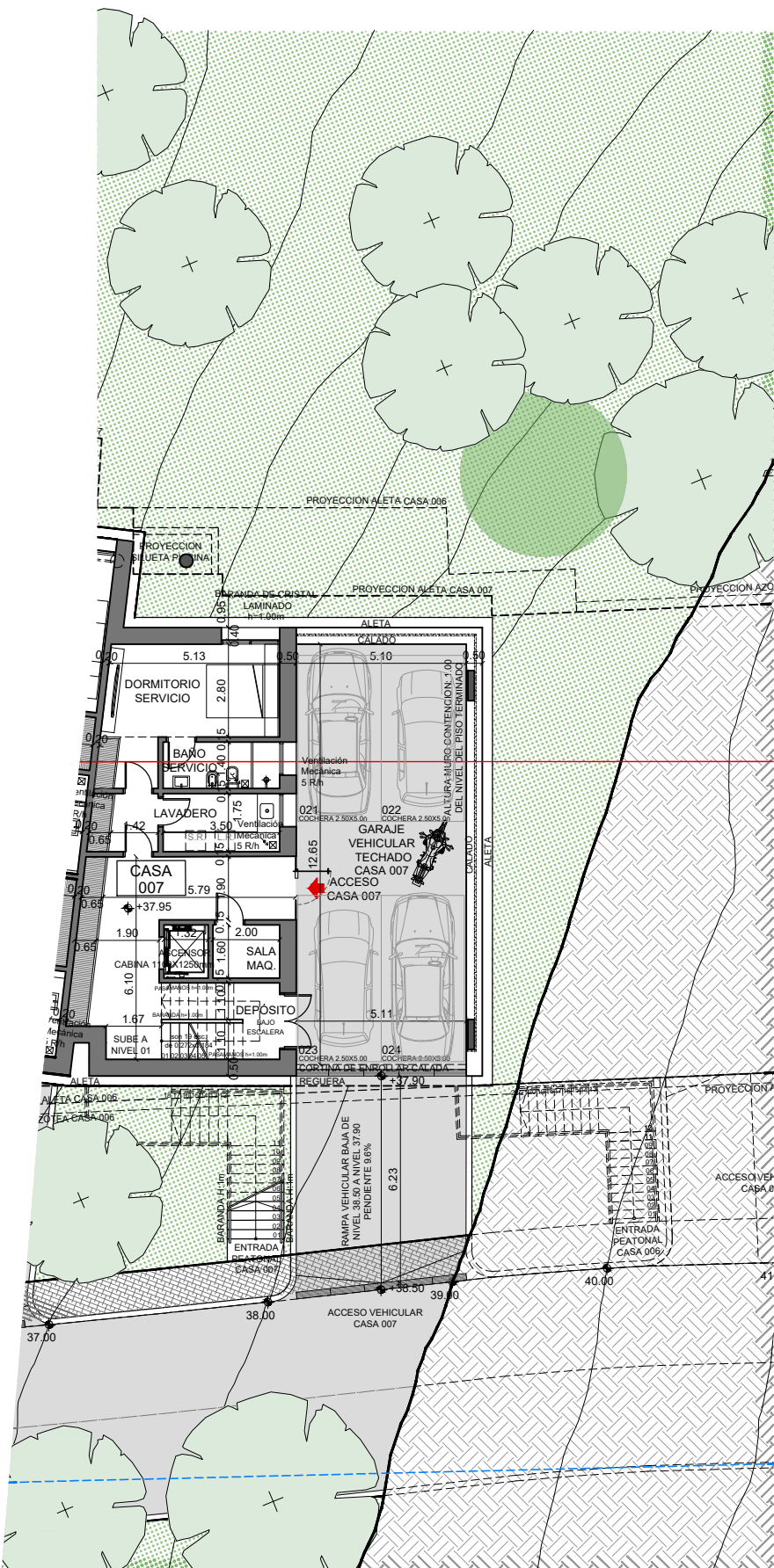
PLANTA NIVEL 01
