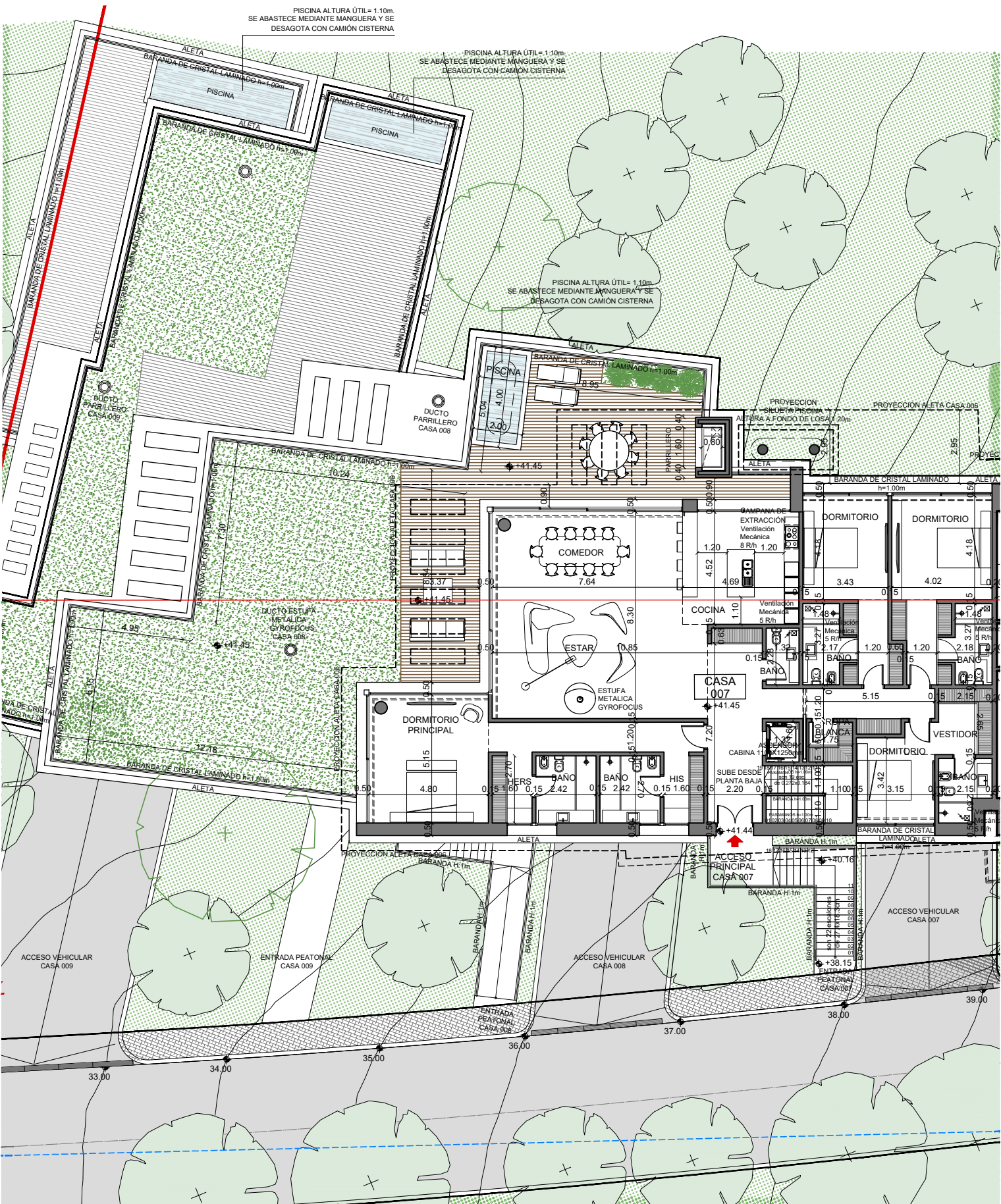
PLANTA NIVEL 02
