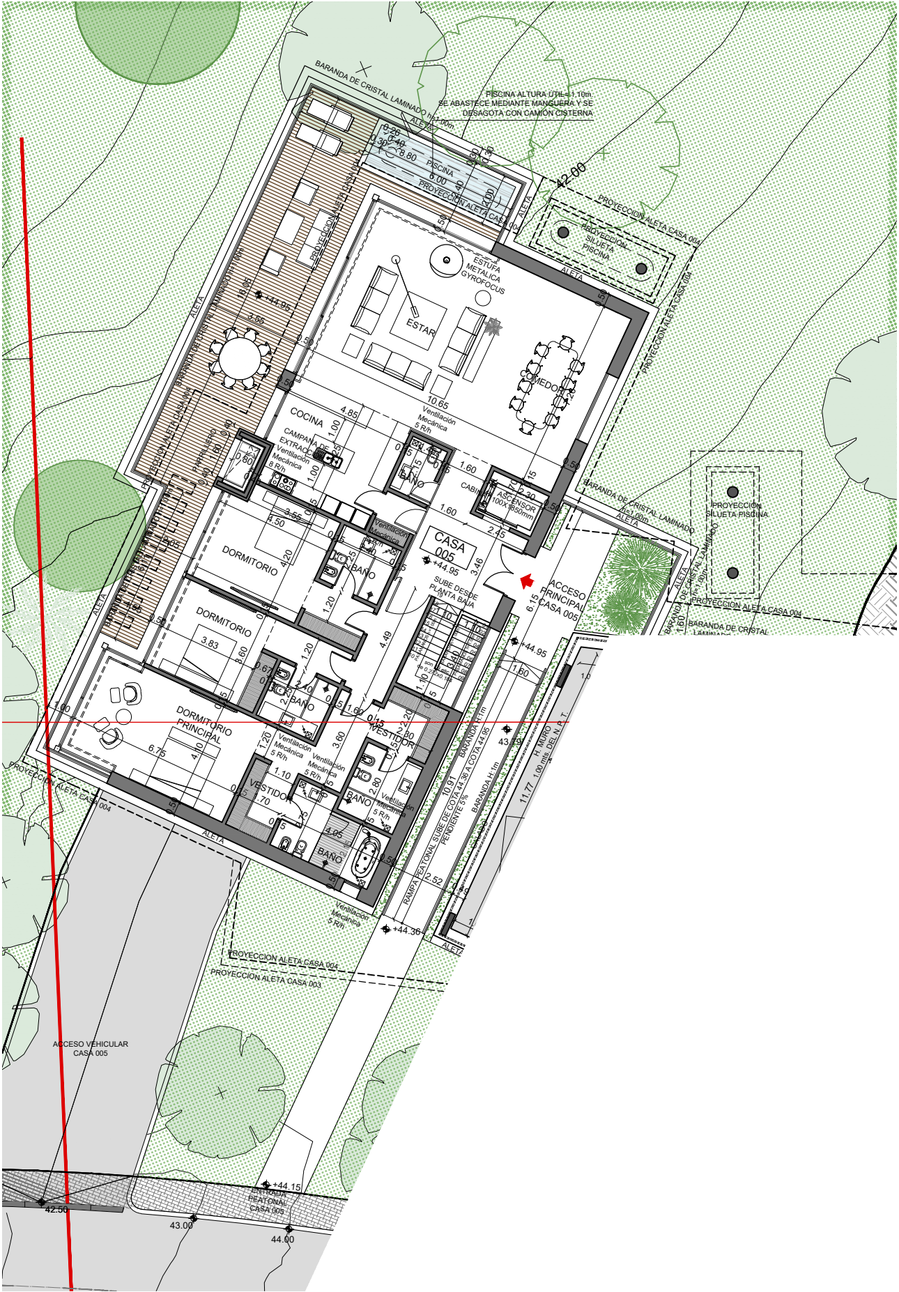
PLANTA NIVEL 02
