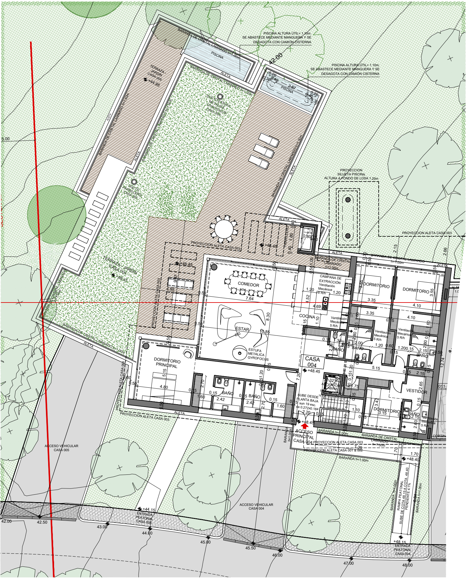
PLANTA NIVEL 02
